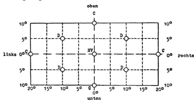
Richtungsdiagramm
